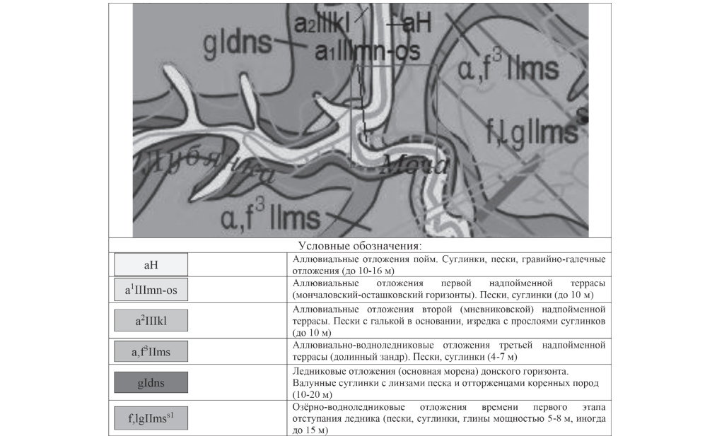
Рис. 1.3.1 Фрагмент карты четвертичных отложений Московской области
