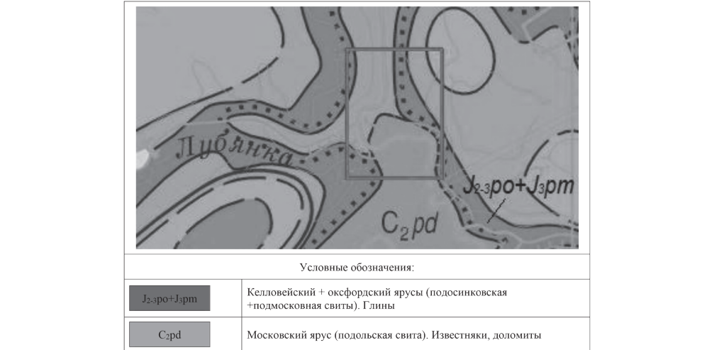
Рис. 1.3.2 Фрагмент карты дочетвертичных отложений Московской области
