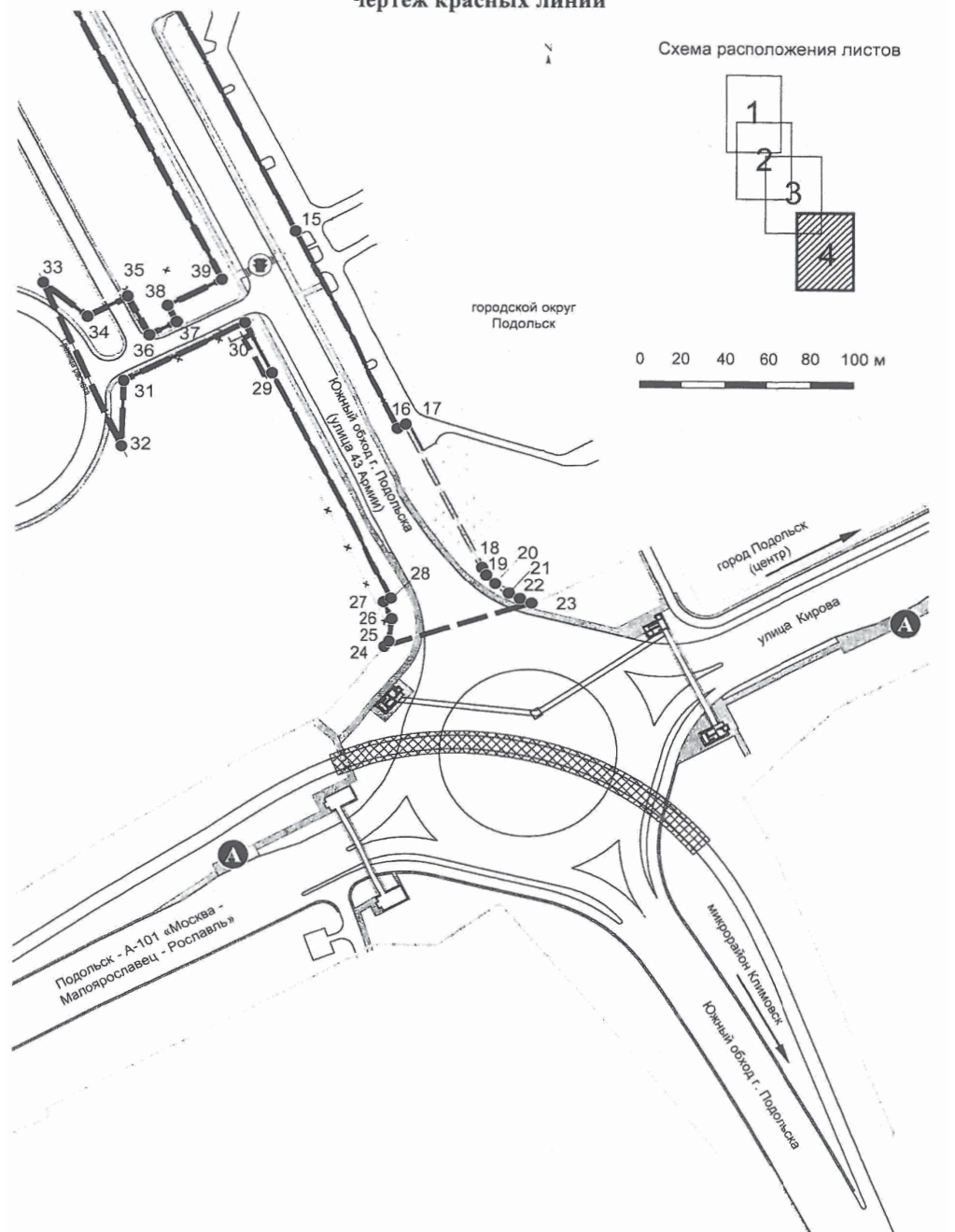
Документация по планировке территории для строительства автомобильной дороги «Южный обход г. Подольска» (улица 43-й Армии) в городском округе Подольск Московской области Чертеж красных линий
