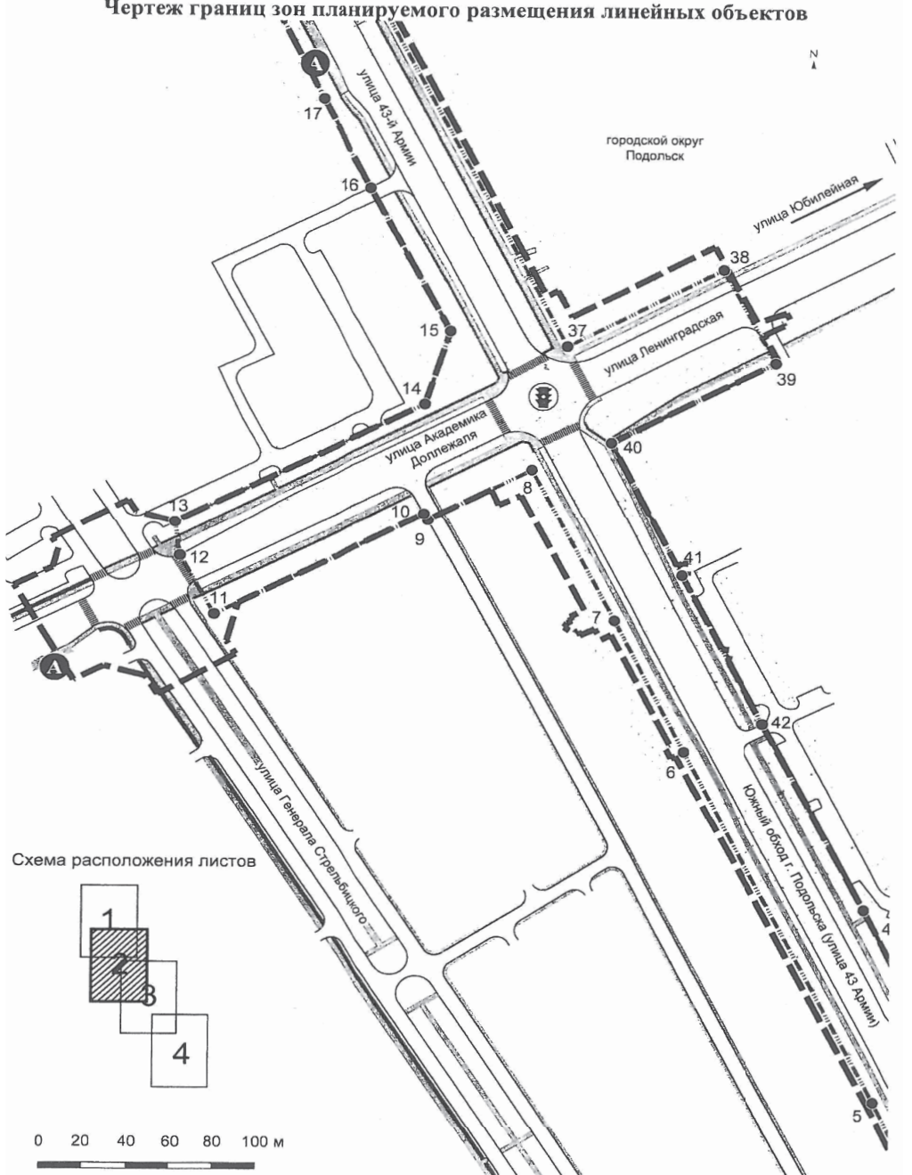
Документация по планировке территории для строительства автомобильной дороги «Южный обход г. Подольска» (улица 43-й Армии) в городском округе Подольск Московской области Чертеж границ зон планируемого размещения линейных объектов
